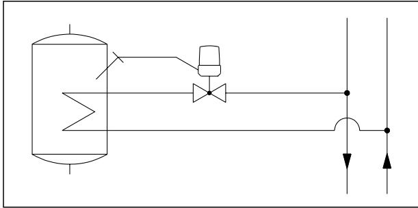
Echauffement d'eau domestique avec réservoir
