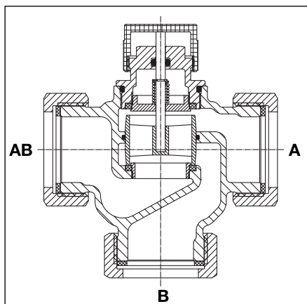
Fig. 5.1 Vue en coupe
