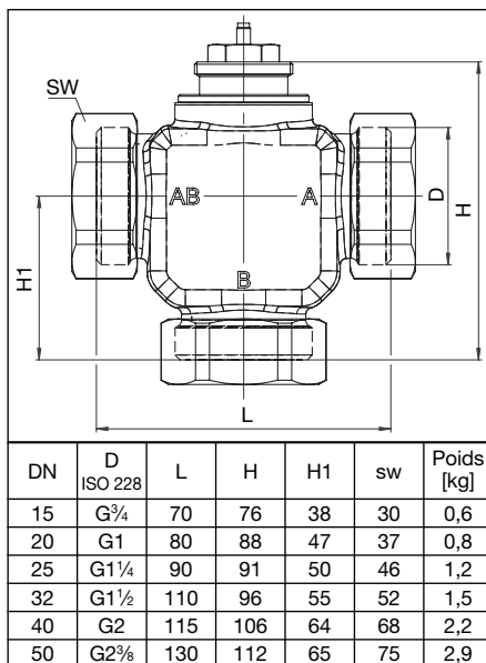
Fig. 4.1 Encombrements
