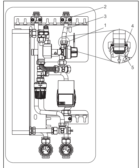
Abb. 5.1 Einbauposition Siebeinsatz
