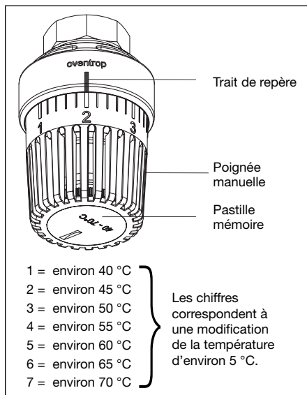
Fig. 6.2 Régulateur de température
