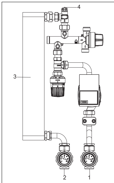
Abb. 6.1 Entlüften „Regumaq XH“
