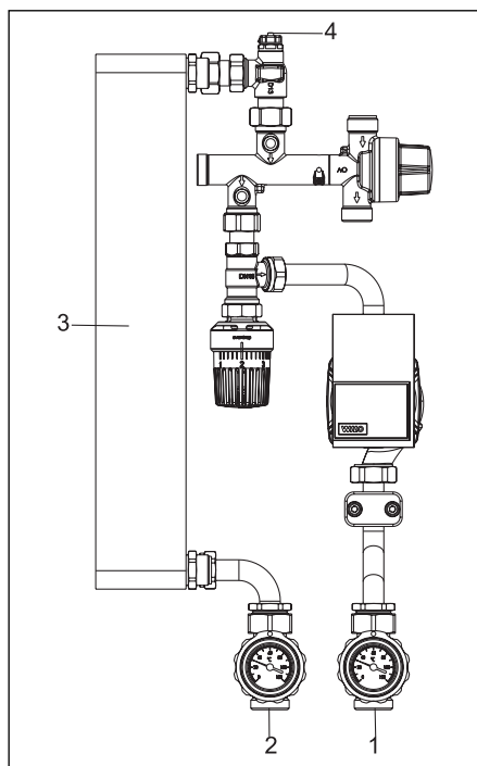
Fig. 6.1 Purge «Regumaq XH»
