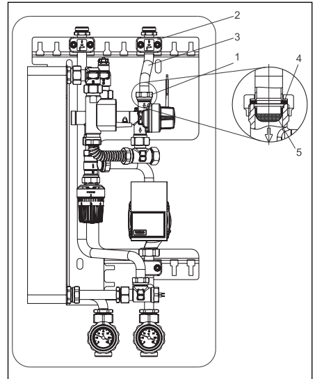
Fig. 5.1 Position de montage du tamis
