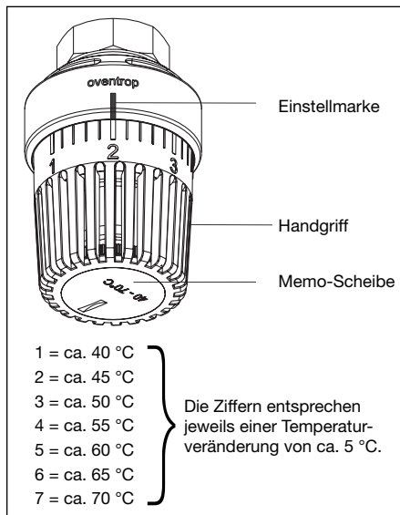
Abb. 6.2 Temperaturregler
