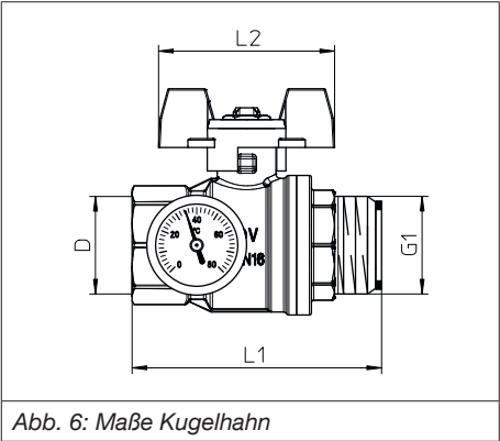
Abb. 6: Maße Kugelhahn
