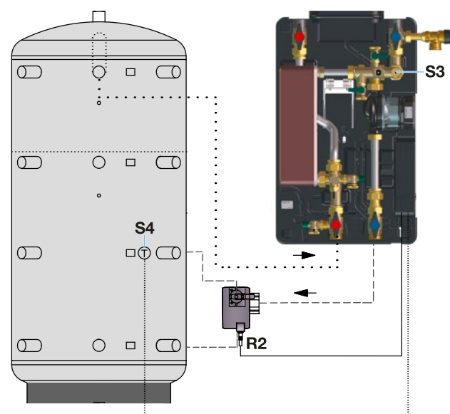
Fig. 26 - Ritorno stratificato
