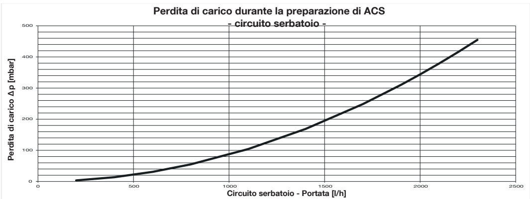
Fig. 37 - Curva caratteristica perdita di carico durante la produzione ACS (circuit serbatoio)
