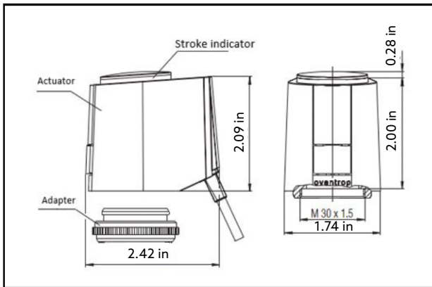
Dimensions
