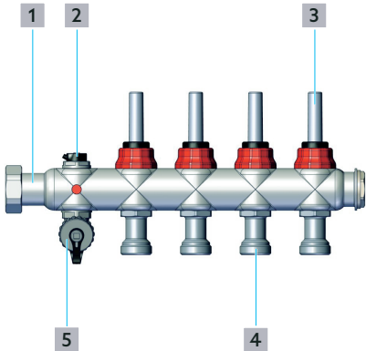
Fig. 1: Aufbau Vorlaufbalken
