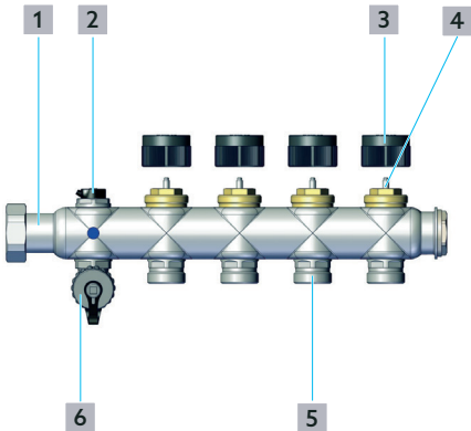
Fig. 2: Aufbau Rücklaufbalken
