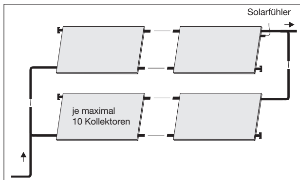
Parallelverschaltung von Kollektorbändern bei V = 35 \text{ l/m}^2\text{h}
