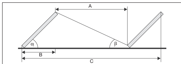
Verschattungsmöglichkeiten
