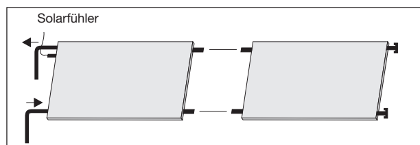
Kollektorband mit einseitigem Anschluss bei V = 35 \text{ l/m}^2\text{h}
