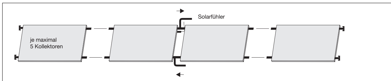
Parallelschaltung von zwei einseitig angeschlossenen Kollektorbändern V = 35 \text{ l/m}^2\text{h}
