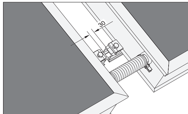
Maßangaben [mm] Kollektor- und Zwischenabstand zur Ermittlung der Feldmaße.
