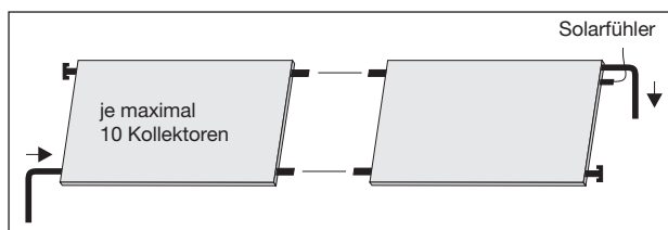
Kollektorband mit wechselseitigem Anschluss, bei V = 35 \text{ l/m}^2\text{h} (spezifischer Volumenstrom)
