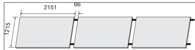
Maßangaben [mm] Kollektor- und Zwischenabstand zur Ermittlung der Feldmaße.
