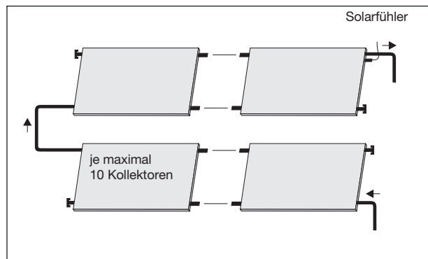
Reihenschaltung von 2 Kollektorbändern bei V = 15 \text{ l/m}^2\text{h} (Low-Flow)
