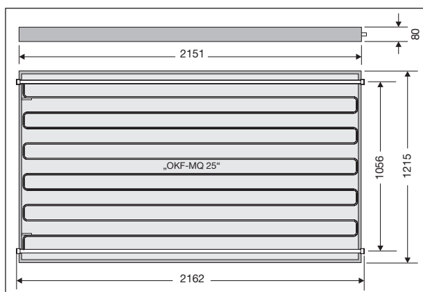
Abmessungen „OKF-MQ25“
