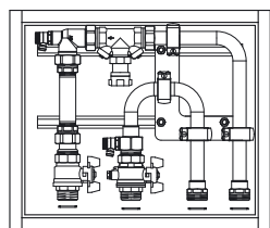
spodní připojení
