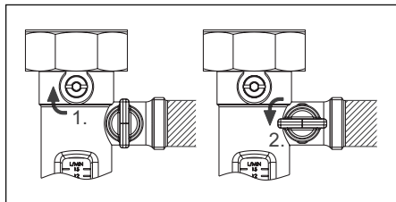
Obr. 6.16 Uzavírací ventil s kulovým kohoutem pro zavírání
