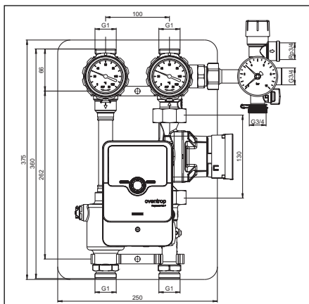
Obr. 4.4 Solární stanice „Regusol ELH-130“ DN 25
