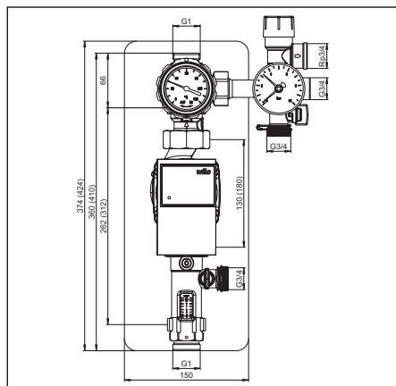
Obr. 4.1 Smyčka čerpadla „Regusol PH-130 (180)“ DN 25
