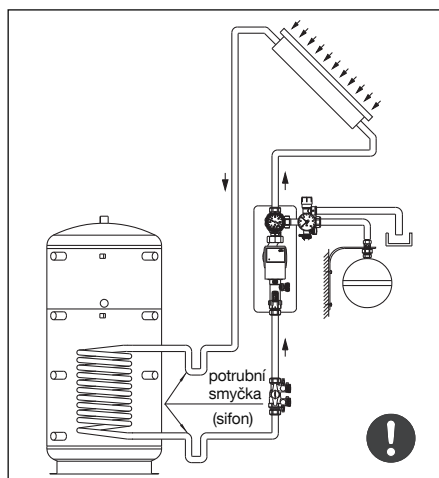
Obr. 6.1 Znáznornění systému
