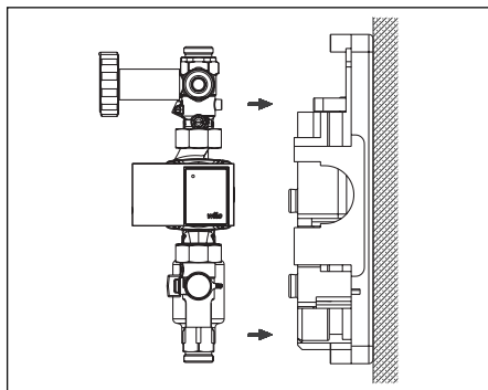
Obr. 6.7 Upevnění stanice
