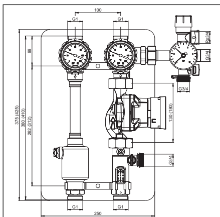
Obr. 4.3 Solární stanice „Regusol LH-130 (180)“ DN 25
