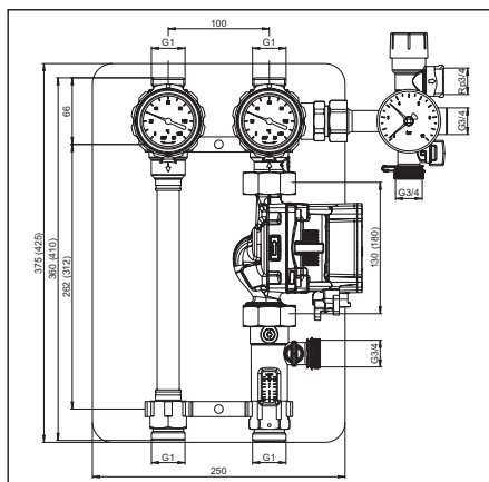
Obr. 4.2 Solární stanice „Regusol SH-130 (180)“ DN 25
