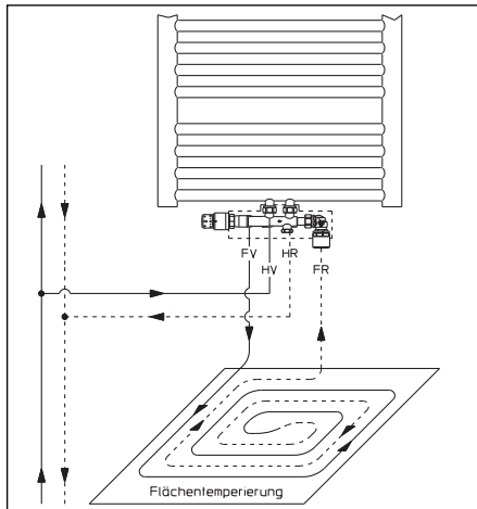
Abb. 5 Anschlussschema
