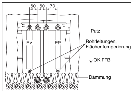
Abb. 9 Wandansicht, Flächenentpermerung
