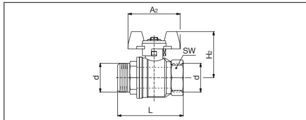
Méretetek, cikkszám: 1076303-10 (DN 10 - DN 32) T- fogantyú fémből (DN 25 Al-ig, DN 32 horganyzott acél)
