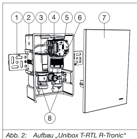
Abb. 2: Aufbau „Unibox T-RTL R-Tronic“
