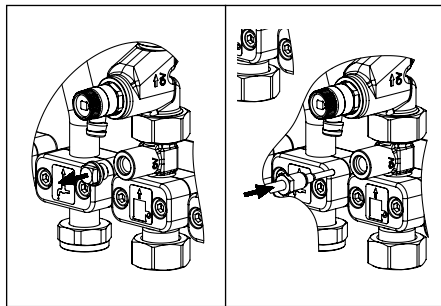
Fig. 6.3 Montaggio tappi
