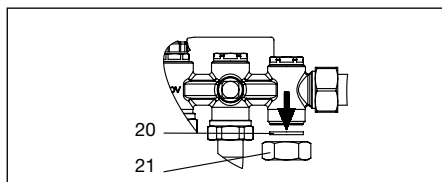
Fig. 6.1 Démontage
