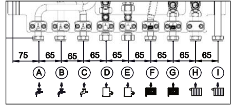
Fig. 4.3 Misure collegamenti
