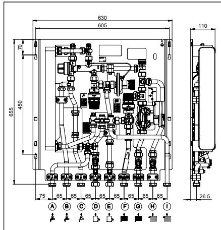
Fig. 4.2 Encombres avec circuit à haute température
