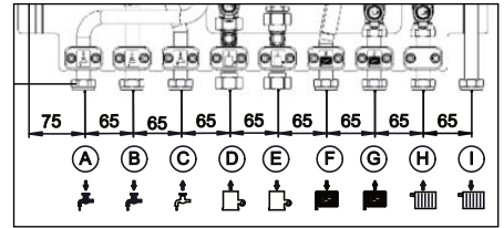
Abb. 4.3 Anschlussmaße
