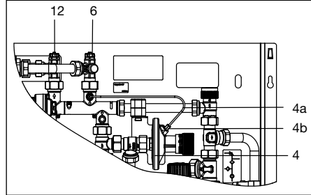
Illustr. 8.2 Bleeding
