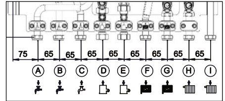
Fig. 4.3 Cotes de raccordement
