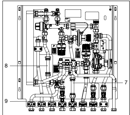
Abb. 6.3 Einbau Kaltwasser- und Wärmezähler
