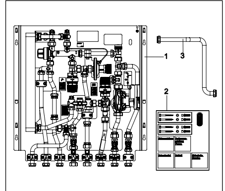
Abb. 3.1 Lieferumfang
