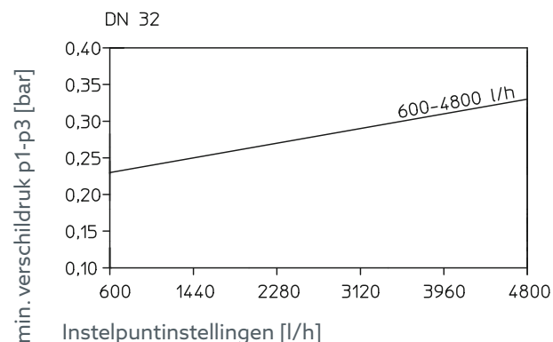
Afb. 13: Minimale verschildrukken
