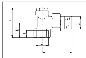
Modèle équerre avec filetage femelle
