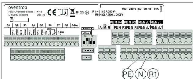
Abb. 12: Zirkulationsset elektrisch anschließen
