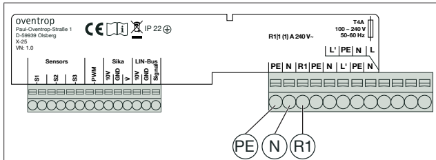
Abb. 11: Zirkulationsset elektrisch anschließen
