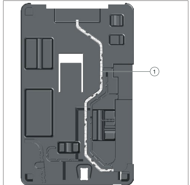
Abb. 13: Kabelführung
