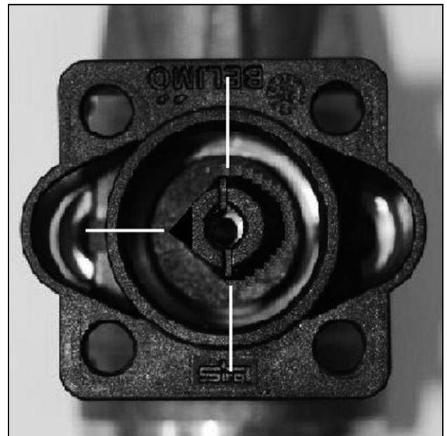
Bild 2: Die Spindel des Kugelhahnes ist nun in Position „offen“ ausgerichtet.
