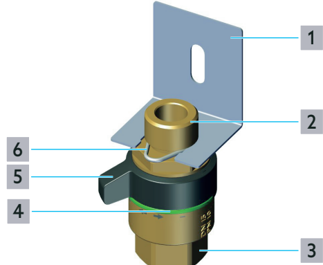
Abb. 2: Aufbau
