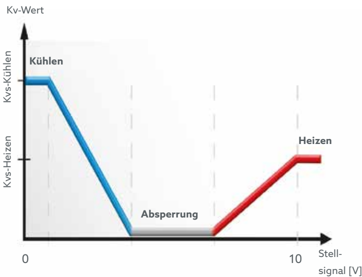
Stellsignal für Heiz- und Kühlbetrieb mit Optibal W6
