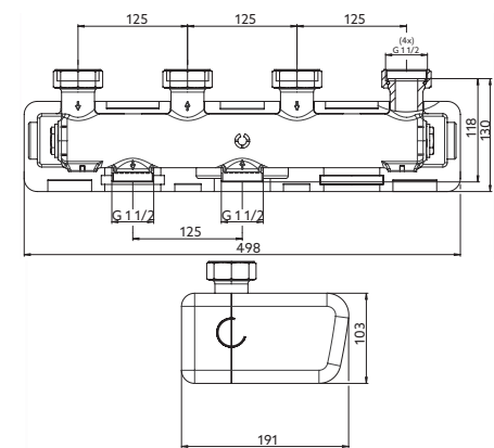
Fig. 2: Encombrements
