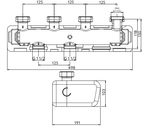
Fig. 2: Dimensions
