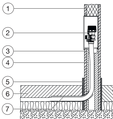
Abb. 6: Einbauquerschnitt
