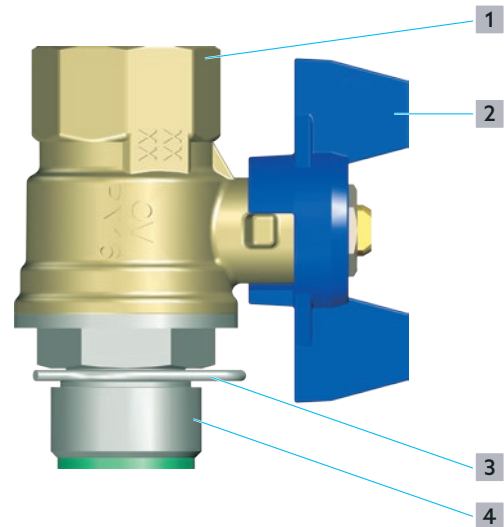
Abb. 3: Aufbau Kugelhahn
