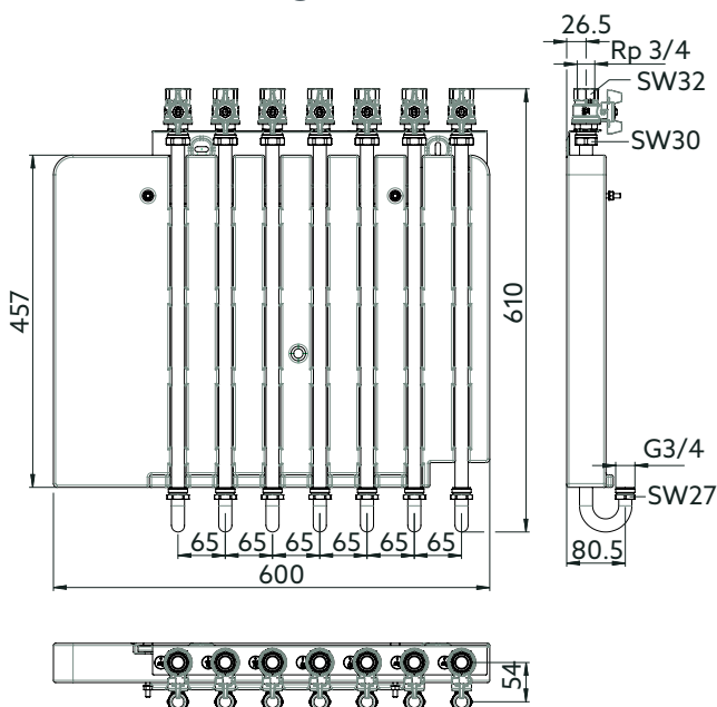
Abb. 2: Abmessungen
