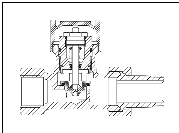
Durchgangsventil
