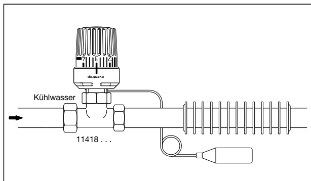
Zweileiter-System Kälte
