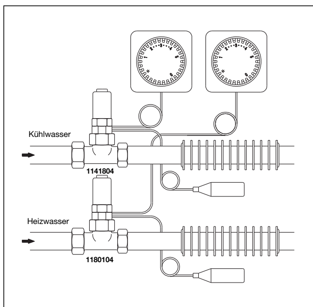
Vierleiter-System 2 Wärmetauscher
