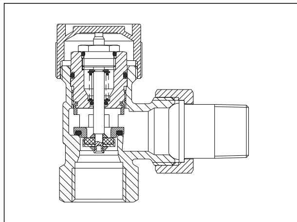
Robinet équerre
