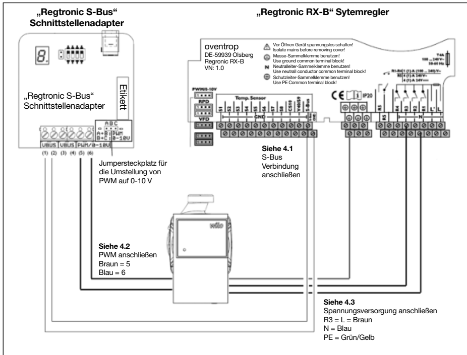
Abb. 5.4 Anschluss-Schema
