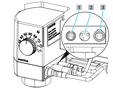
Abb. 5: Steckverbindungen
