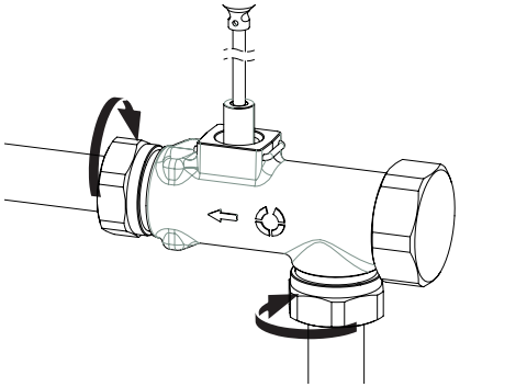
Abb. 4: Volumenstromsensor demontieren
