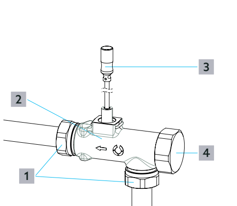
Abb. 1: Aufbau
