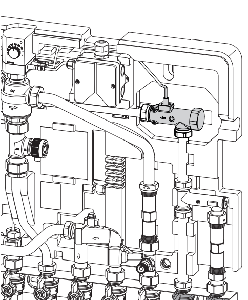
Abb. 2: Position in der Wohnungsstation Regudis W-HTE
