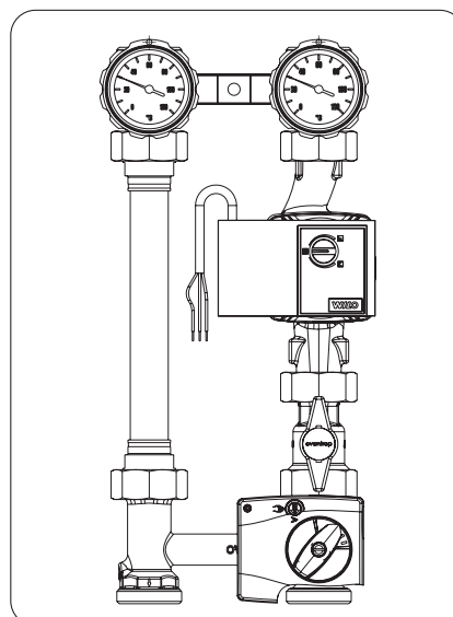
Regumat M3-180 avec robinet d'isolement à tournant sphérique
