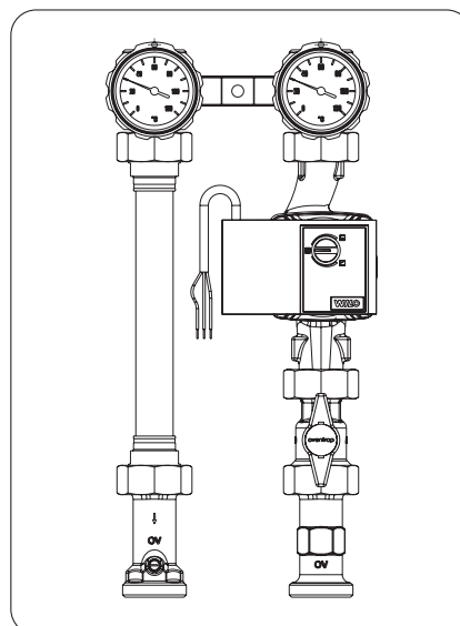
Regumat S-180 avec robinet d'isolement à tournant sphérique
