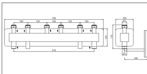
Dimensioni collettore DN 20, 3 circuiti
