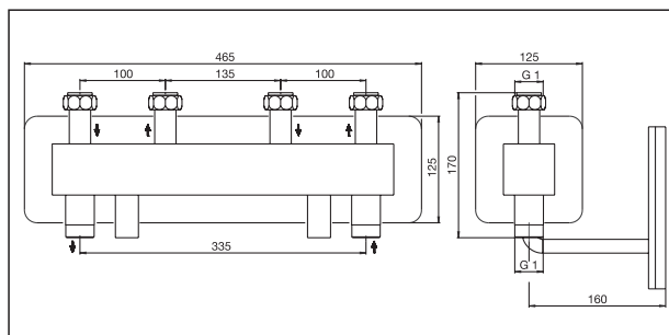
Dimensioni collettore DN 20, 2 circuiti
