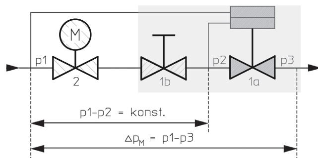
Fig. 3 - Principio di funzionamento di "Cocon QTZ", PN25
