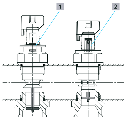
Fig. 5: Einstellung Durchflussindikator
