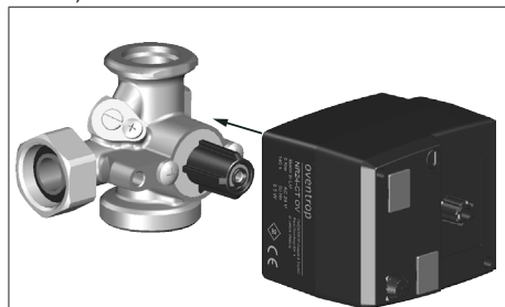
Abb. 4: Montage du moteur
