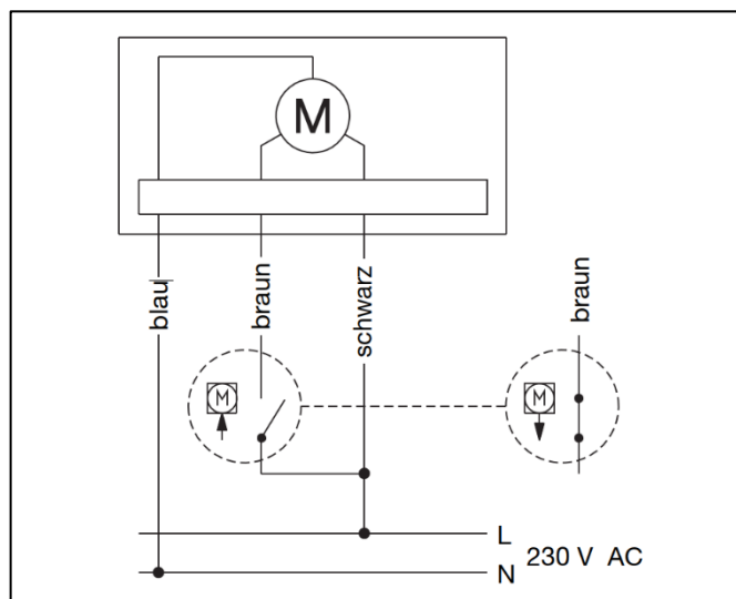
Schakelschema
