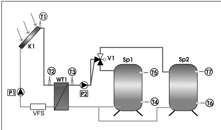
„Regusol X-Duo” - Încărcarea a 2 boilere
