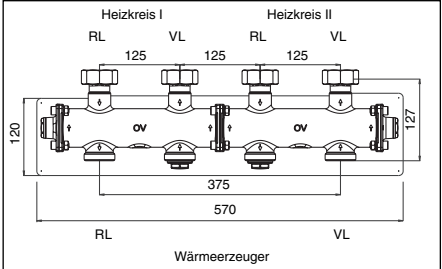
Modulverteiler für 2 Heizkreise
