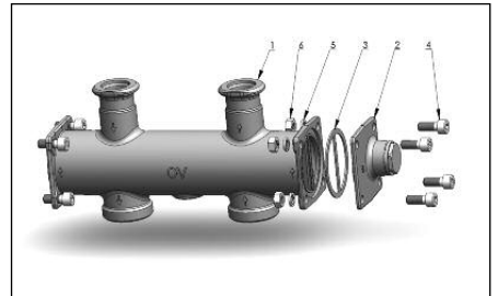
Einbau des Erweiterungsmoduls
