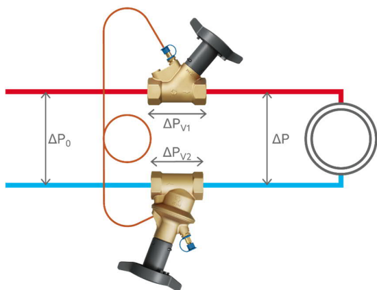
Schemat ideowy
