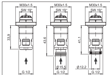
Fig. 1: Dimensions et sens de circulation type GHQ
