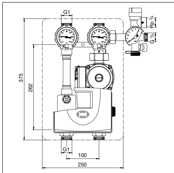
„Regusol EL-130” – moduł dwupionowy
