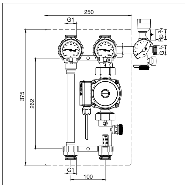
„Regusol-130” – moduł dwupionowy
