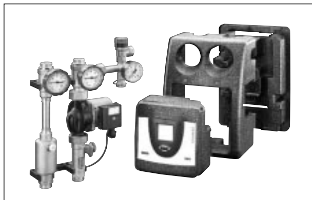
„Regusol E-130” – moduł dwupionowy
