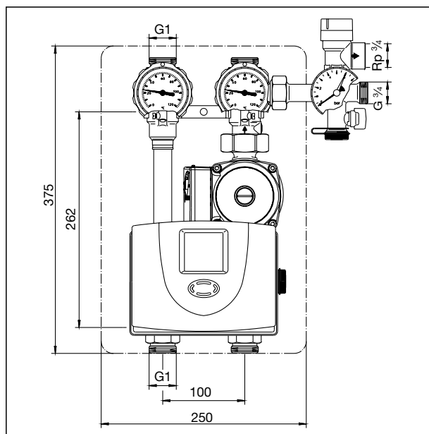
„Regusol E-130” – moduł dwupionowy
