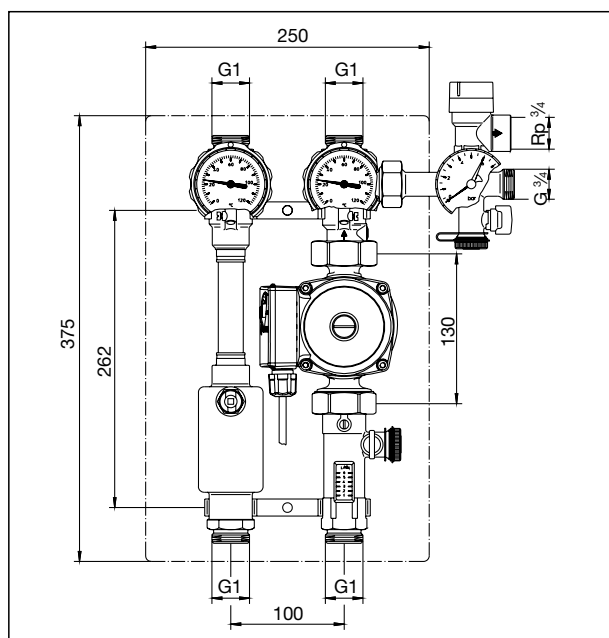
„Regusol L-130” – moduł dwupionowy
