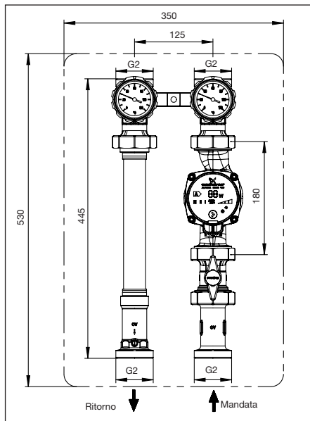
Gruppo pompa "Regumat S-180"
