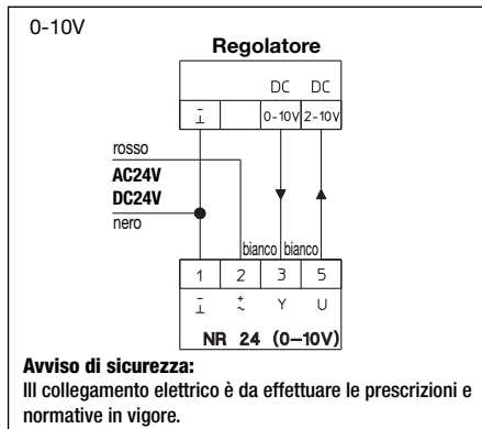
Schema di collegamento elettrico
