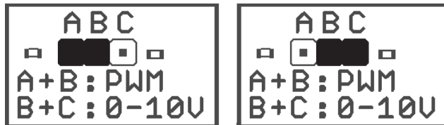
Jumperstellung für PWM-Signal
