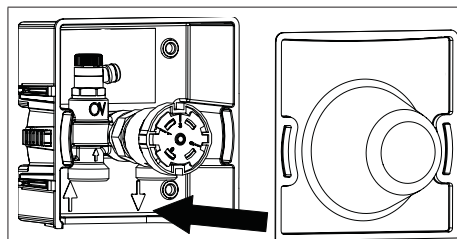
Abb. 12: Bauabdeckung aufsetzen
