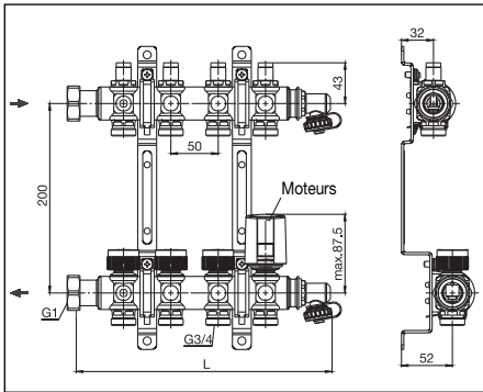
Fig. 1: Encombrements
