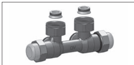
Abb. 2 Anschlussarmatur „Multiflex FQ“, Eck, Linksan- schluss, G ¾ ÜM x G ¾ AG
