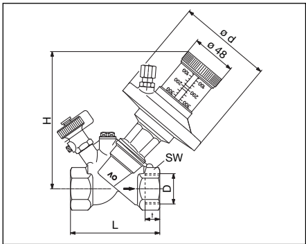
Fig. 2: Regolatore tipo 10645/4704-16 e 1664706-16 entrambe i lati FF secondo EN 10226
