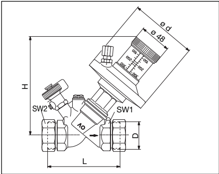
Fig. 3: Regolatore tipo 106 46/48 04-16 entrambe i lati FM e calotte
