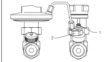
Illustr. 6.1: «Hycoco DTZ» Illustration du raccordement de la ligne d'impulsion, montage sur le retour
