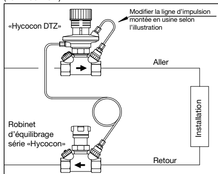
Illustr. 6.3: «Hycoco DTZ» Montage sur l'aller (seulement DN 32 + 40)
