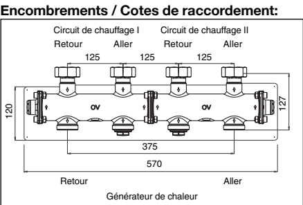
Module de distribution pour 2 circuits de chauffage
