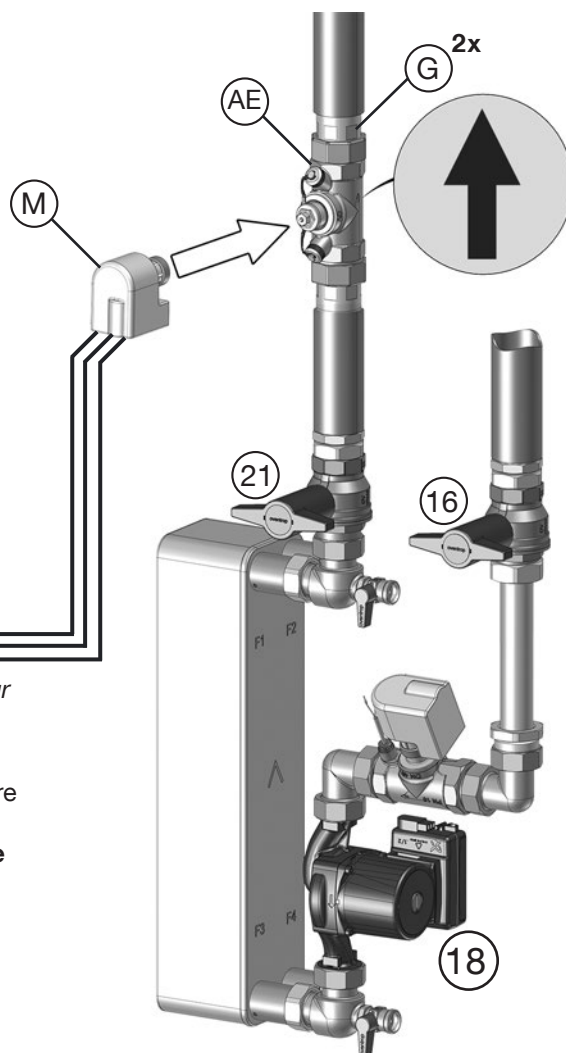
Fig. 4.12: Montage du dispositif d'arrêt et du moteur
