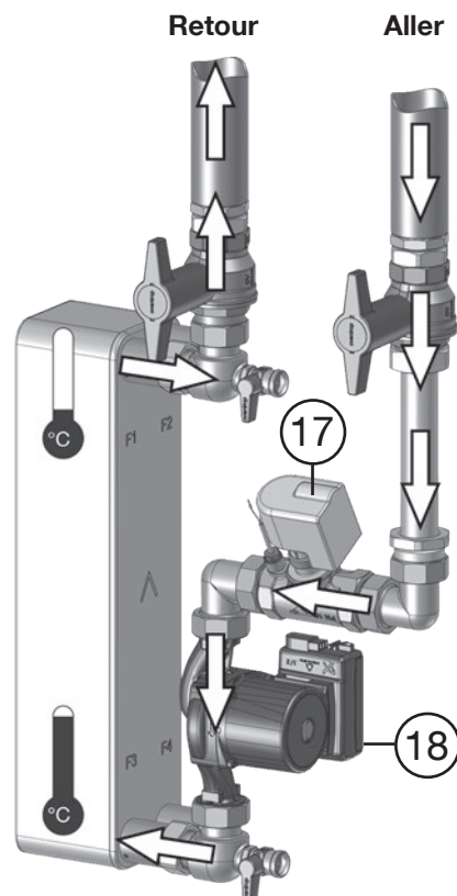
Fig. 3.2: Côté circuit primaire avec l'aller venant du ballon tampon et le retour vers le ballon tampon
