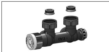
Obr.2 Připojovací armatura "Multiblock T", rohové provedení \frac{3}{4} PM x G \frac{3}{4} AG
