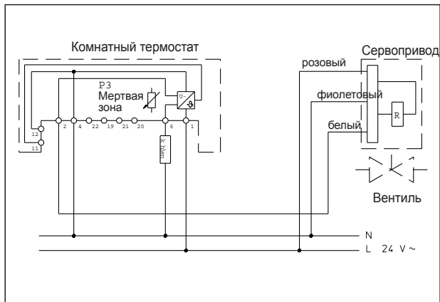
Схема переключения
