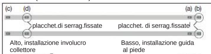
Illustr. 5: guide di montaggio pre-assemblate per "installazione sul tetto" (a) e "installazione al piede" (b)
